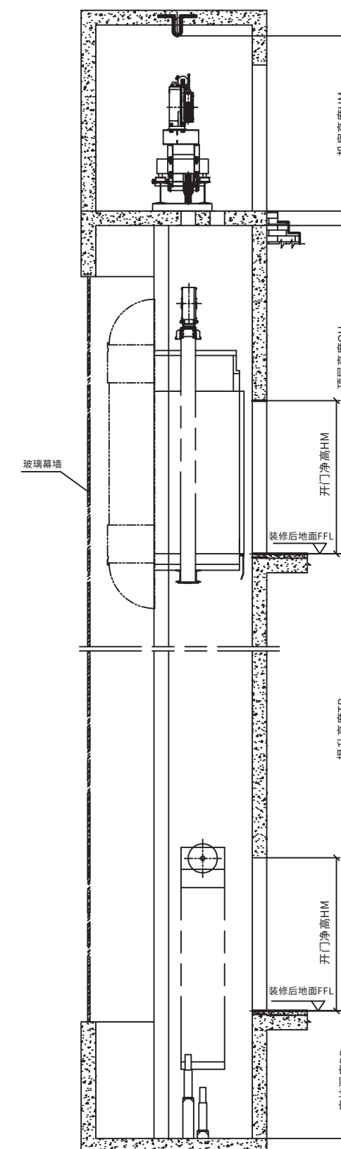
井道纵剖面图 shaft section plan
